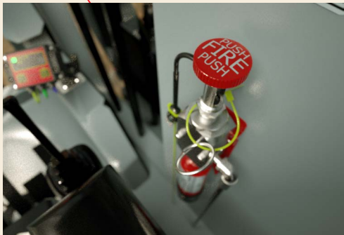
Manual Actuator
